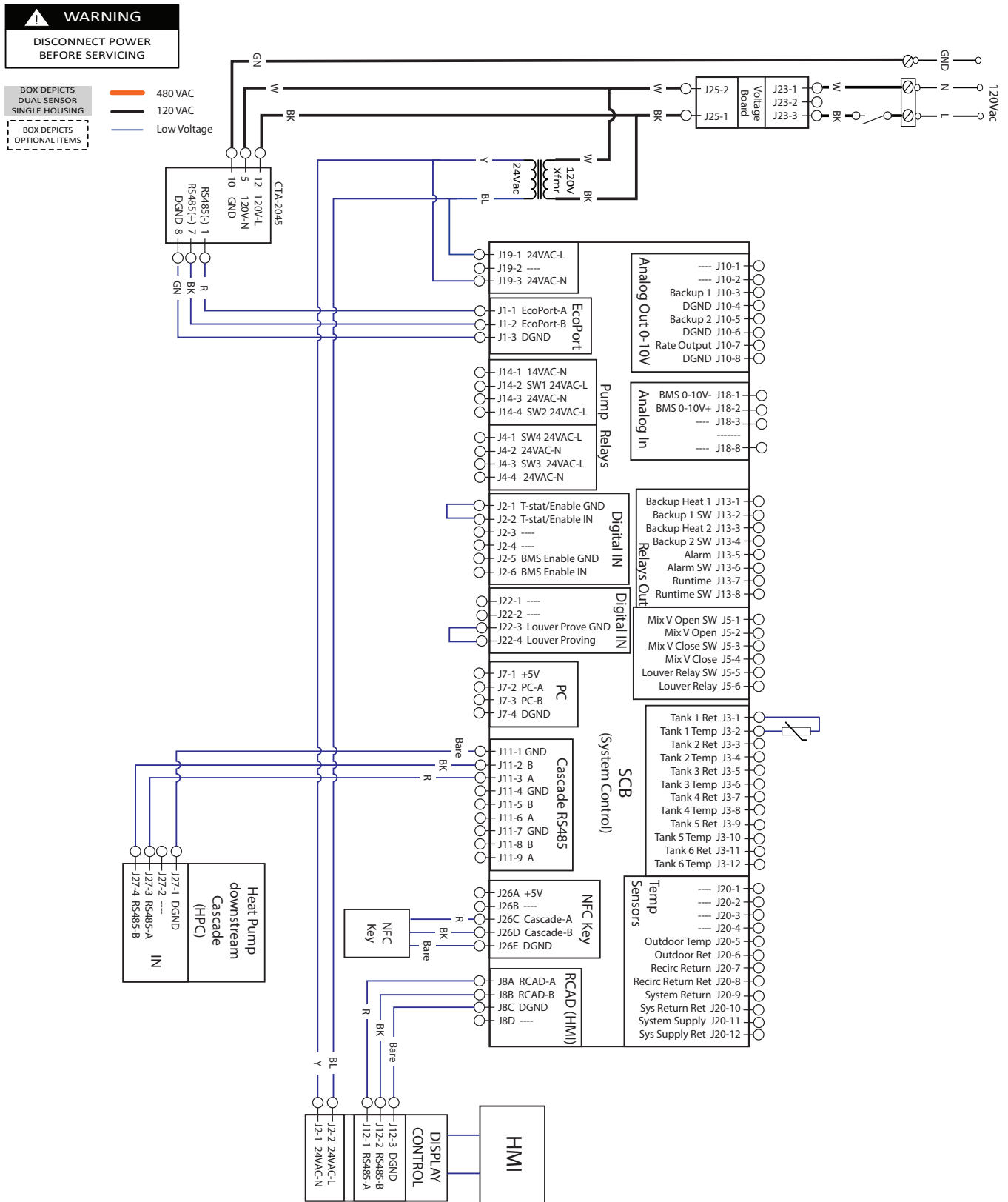
Figure 12-5 Schéma de câblage du panneau d'affichage
